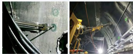
隧道襯砌岩栓加固
