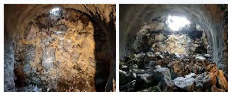
隧道開挖崩積層抽坍
