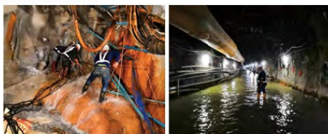
暗挖隧道湧水
